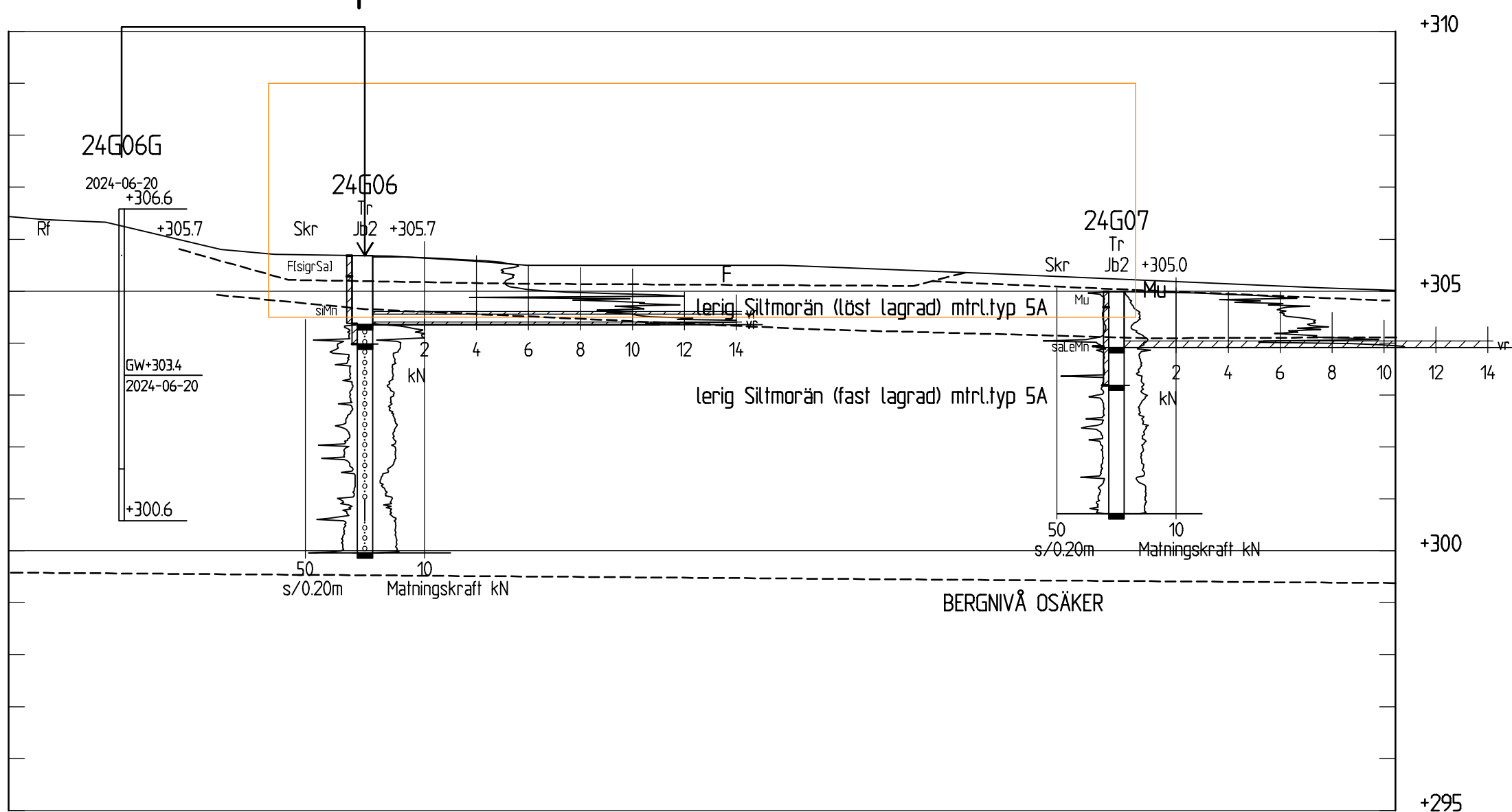
SEKTION C-C - VID PLANERAD BYGGNAD 1: 100
